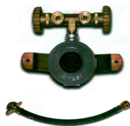
Gasna rampa sa 2 gumena creva
